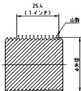
ねじ断面
