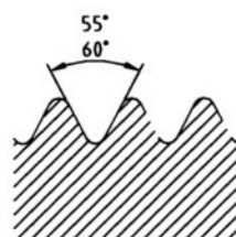
ねじ山角度
